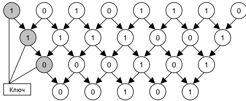
Рис. 3. Шифрование с генерацией ключа
