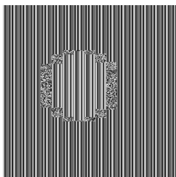
Рис. 9. Метод RIJNDAEL
