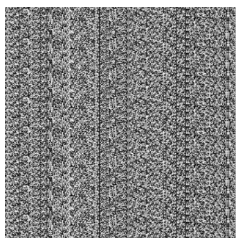
Рис. 10. Метод SEA
