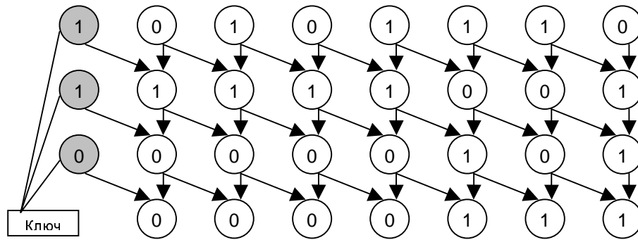
Рис. 4. Шифрование с фиксированным ключом
