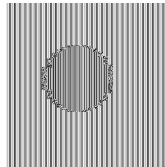
Рис. 6. Метод 3DES
