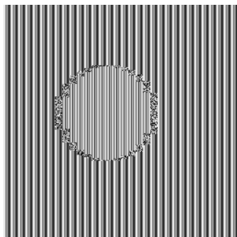
Рис. 7. Метод DES
