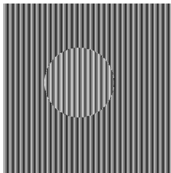
Рис. 8. Метод BLOWFISH
